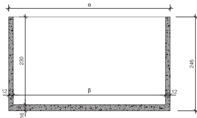
Langdoorsnede
