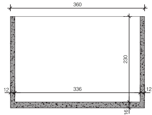
Dwarsdoorsnede
