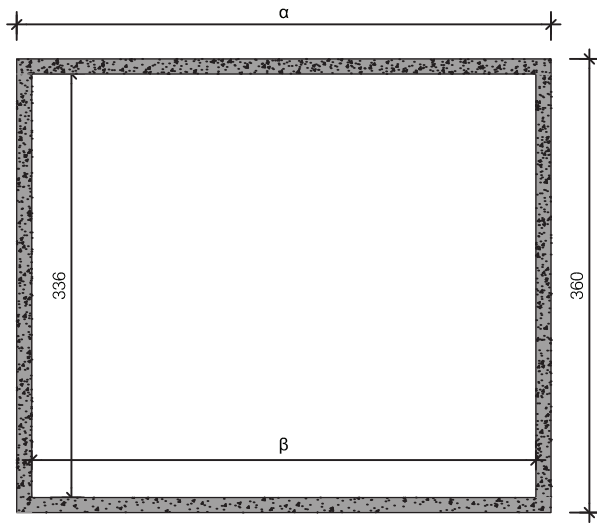
Doorsnede
